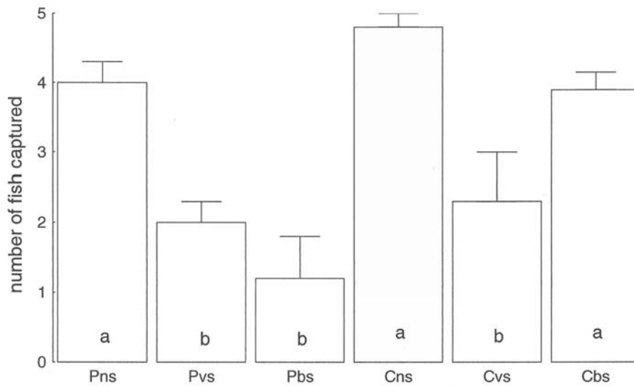
Figure 1. Number (mean of five replicates \pm 1 SE) of fish captured during 21 hours by largemouth bass in tanks simulating different structure types. P-pumpkinseed, and C-Cyprinid, whereas ns-no structure, vs-vegetation structure and bs-bottom structure. Letters for prey and structure types are combined to represent a particular treatment. Bars within a prey type followed by the same letter are not significantly different (post-ANOVA Tukey HSD, p > 0.05 ). Número de peces (media de cinco replicas \pm 1 SE) capturados durante 21 horas por los black bass en los tanques simulando diferentes tipos de estructuras. P-caladinos, y C-ciprinidos, mientras que ns-sin estructura, vs-estructura con vegetación y bs-estructura en el fondo. Las letras para las presas y el tipo de estructuras estan combinadas para presentar un determinado tipo de tratamiento. Las barras dentro de un tipo de seguidas de la misma letra no son significativamente diferentes (a partir de un ANOVA Tukey HSD, p > 0.05 ).
